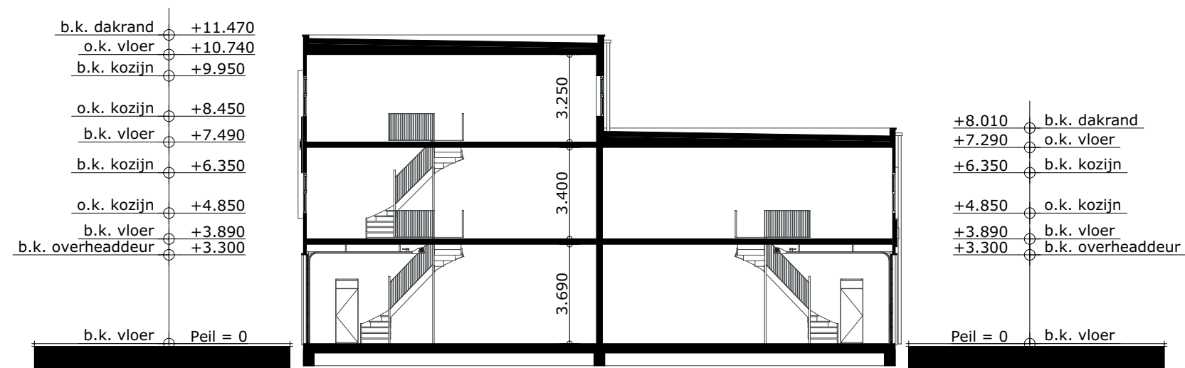
DOORSNEDE B-B
