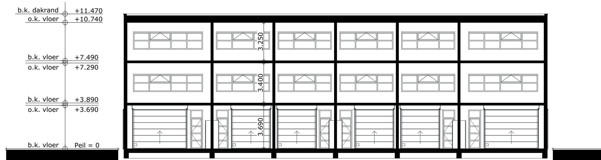
DOORSNEDE A-A
