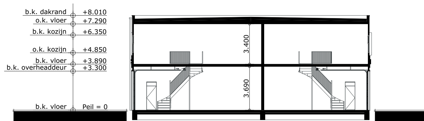
DOORSNEDE B-B
